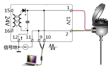
图 9 配电-输入-输出三隔离配置
