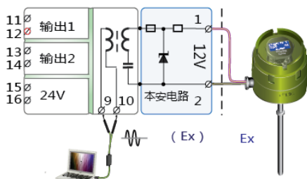
图 11 通用 HART 通讯配电隔离器或配电隔离安全栅
