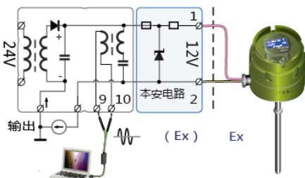
图 10 本安和三隔离配置原理图
