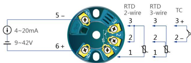
图 2 端子接线图
