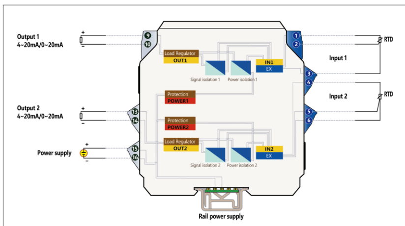
2 入 2 出 热电阻输入安全栅 框图/接线图 (适用于：型号 TCA-RTD22)
