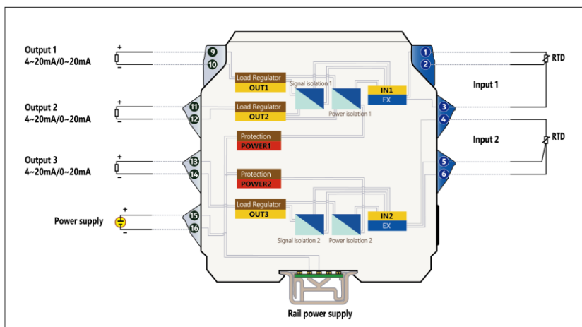
2 入 3 出 热电阻输入安全栅 框图/接线图 (适用于：型号 TCA-RTD23)
