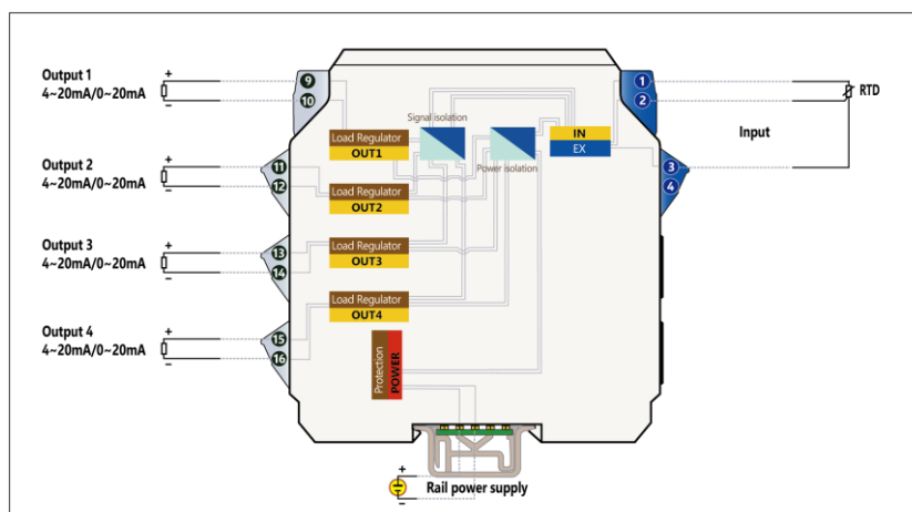
1 入 4 出 热电阻输入安全栅 框图/接线图 (适用于：型号 TCA-RTD14)
