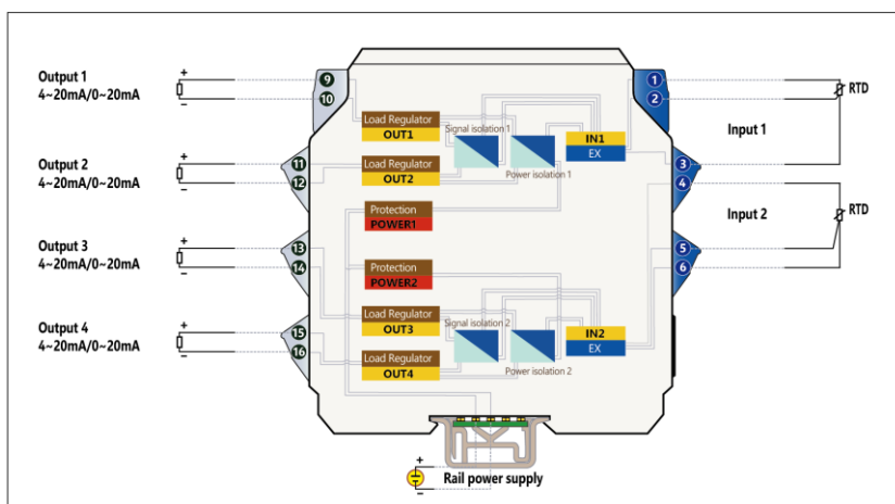
2 入 4 出 热电阻输入安全栅 框图/接线图 (适用于：型号 TCA-RTD24)
