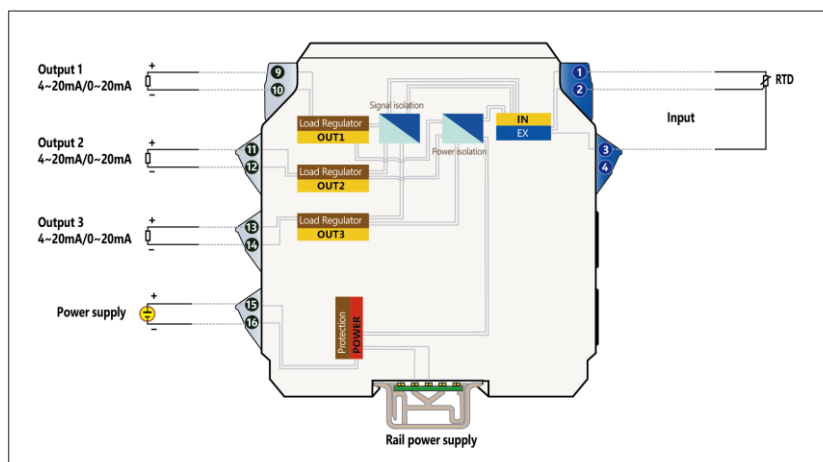
1 入 3 出 热电阻输入安全栅 框图/接线图 (适用于：型号 TCA-RTD13)
