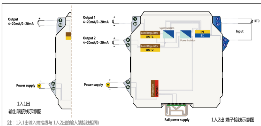
1 入 1 出/1 入 2 出 热电阻输入安全栅 框图/接线图 (适用于：型号 TCA-RTD11, TCA-RTD12)
